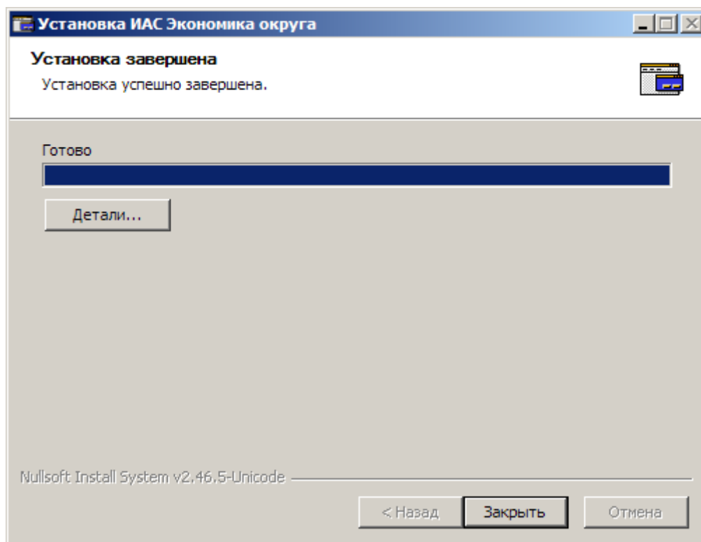
Рисунок 5 Завершение установки
